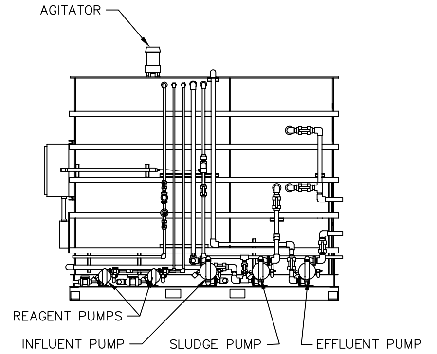
RIGHT ELEVATION
